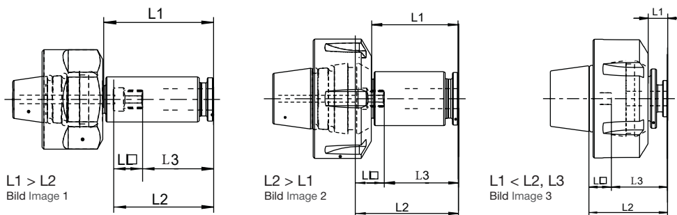
Synchroaufnahme STL Synchro location STL
