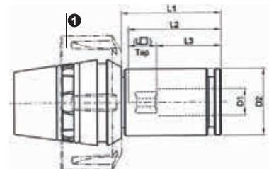
Synchroeinsatz STA Synchro adaptor STA
