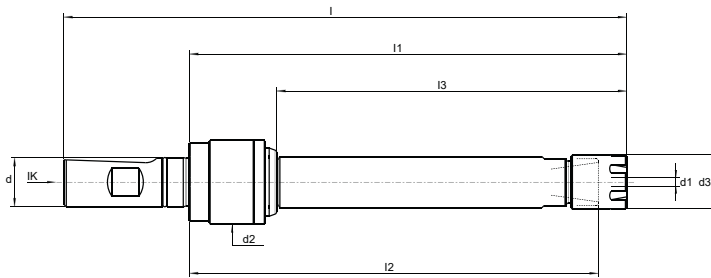
S3D1-ER16M-K1-W20 - DIN1835 Form B und E
